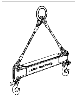
Figura 14. Balancín
